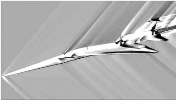
X-59 验证机激波模拟图像
