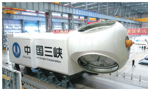
在福建三峡海上风电国际产业园下线的16兆瓦海上风电机组(新华社/图)
