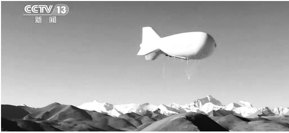
2022年“巅峰使命”珠峰科考中,我国科学家用浮空艇进行大气科学观测,最高升空至9050米
