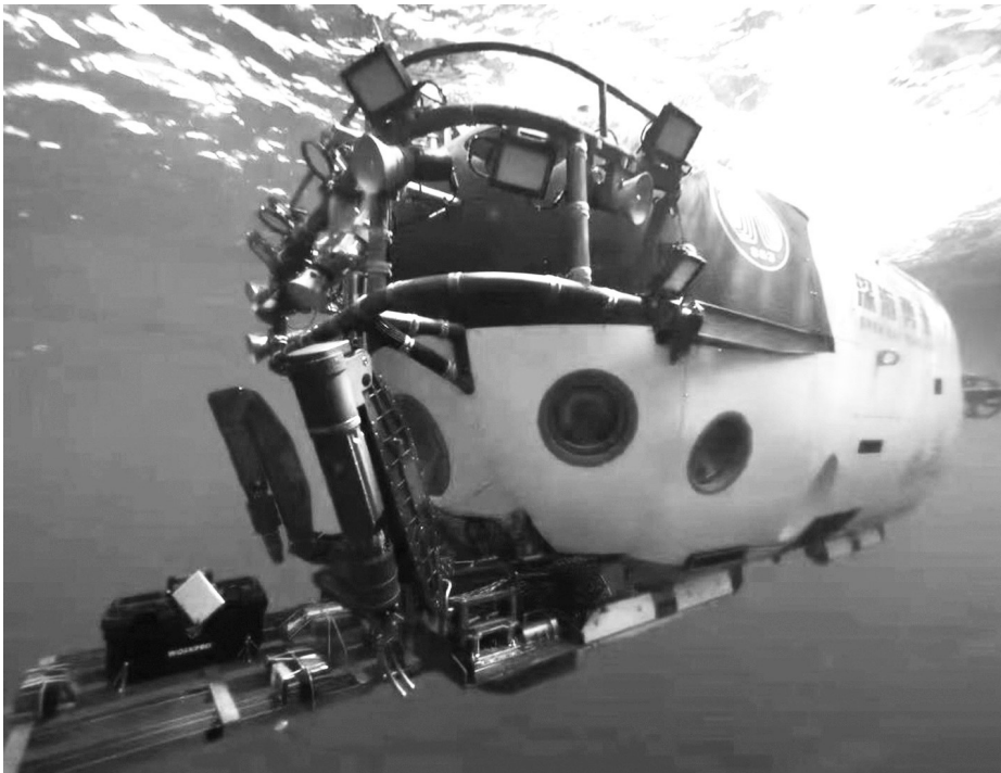
“深海勇士号”载人潜水器
