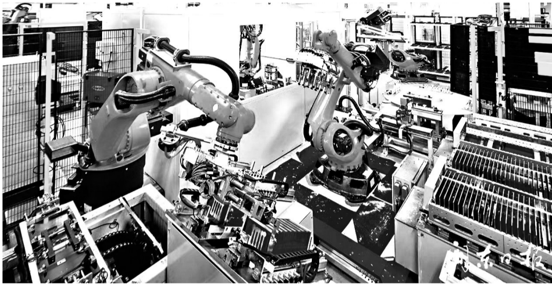
电池模组生产(宁德时代图) 宁德时代新能源科技有限公司自动化
