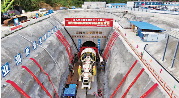
TBM盾构机开挖
