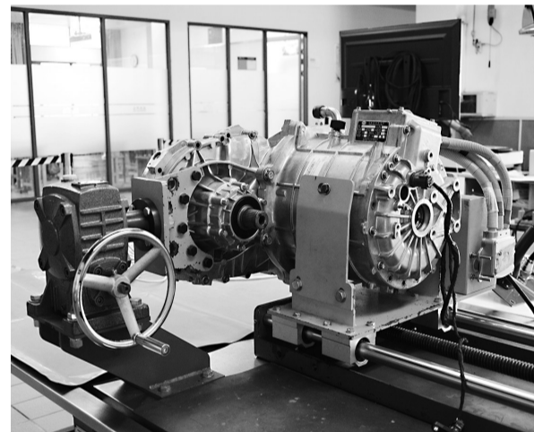
福建工业学校驱动电机拆装与检测训练平台
