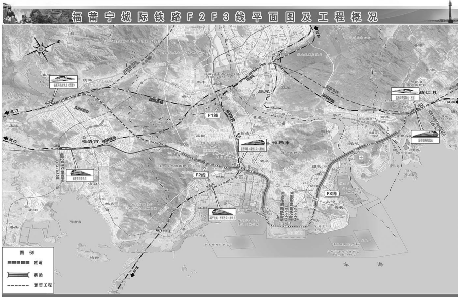
福莆宁F2、F3线路初步设计走向图
