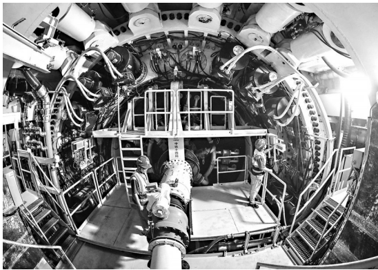
盾构机内部
